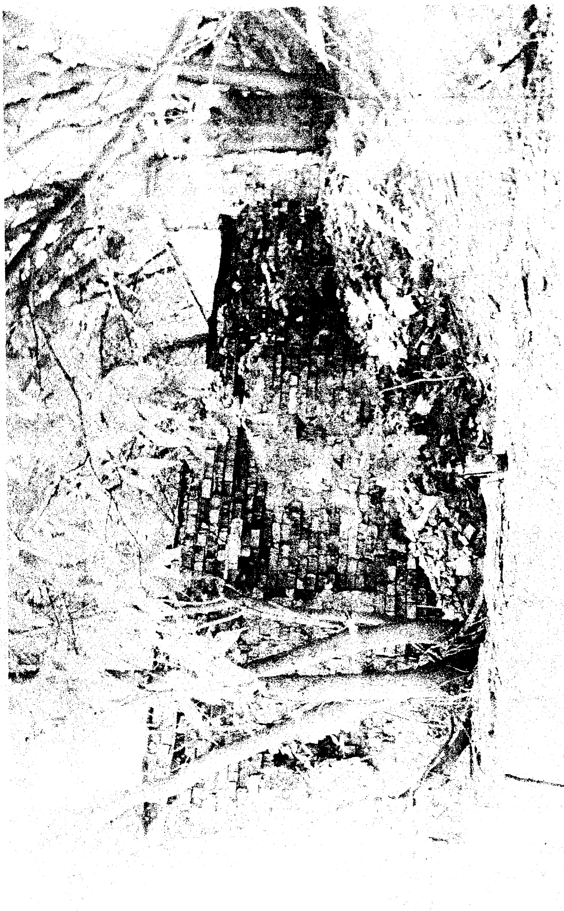
Фото 3. Фасад по осі «1», будівля вписана в схил. Спостерігається розшарування кладки стіни на глибину 15-20см.
