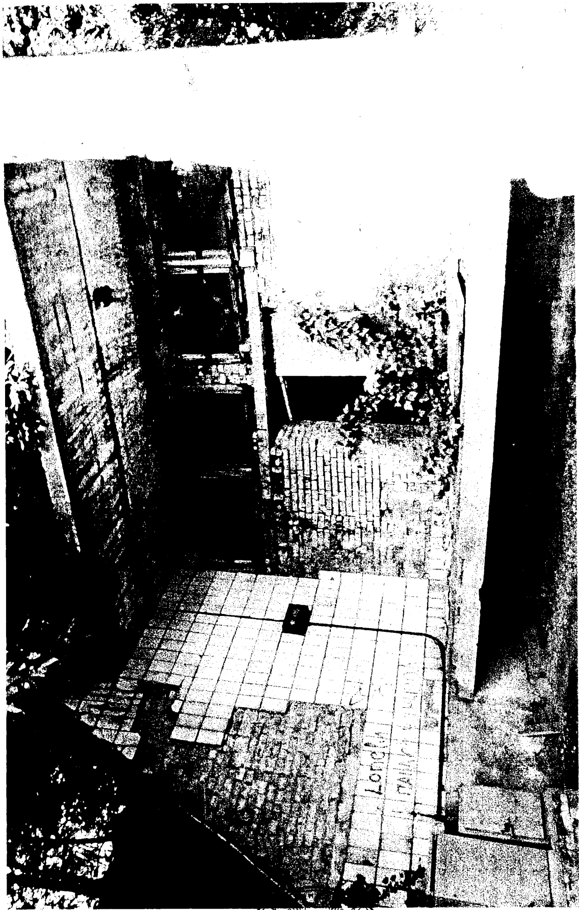
ФОТО 2. Стіна по осі «2». Ліворуч від дверного отвору спостерігається вертикальна тріщина з шириною розкриття 30мм, випадання цеглин та розчину з кладки.
